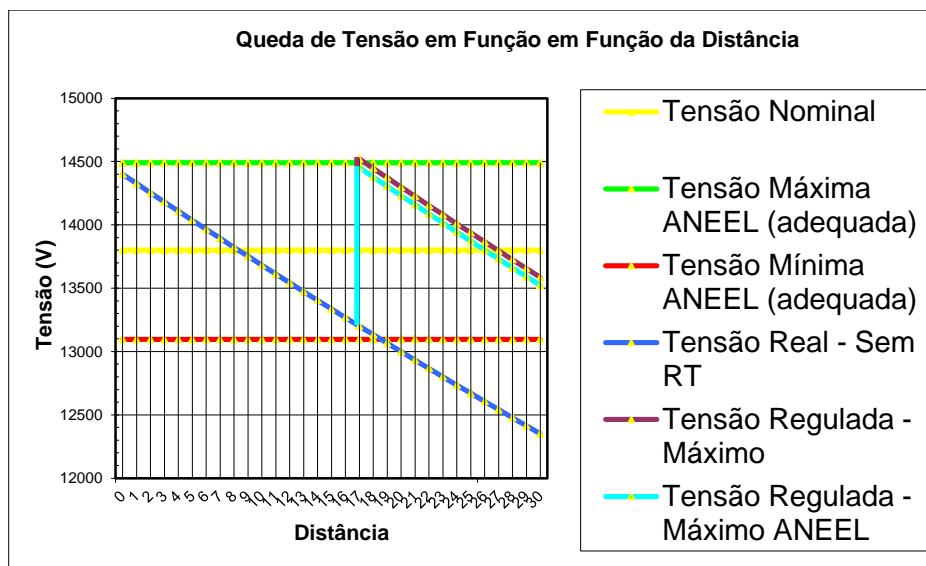
Figura 1 - Gráfico da queda de tensão. Fonte: CEMIG (2002)
